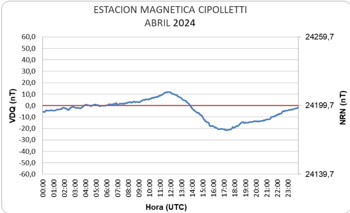
Figura 7: Variación Diaria Calma del mes de abril
