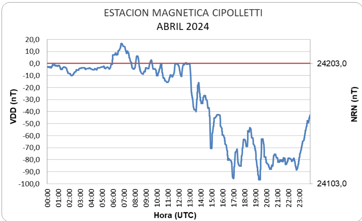
Figura 8: Variación Diaria Perturbada del mes de abril
